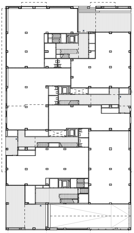
0 10 Planta baixa
