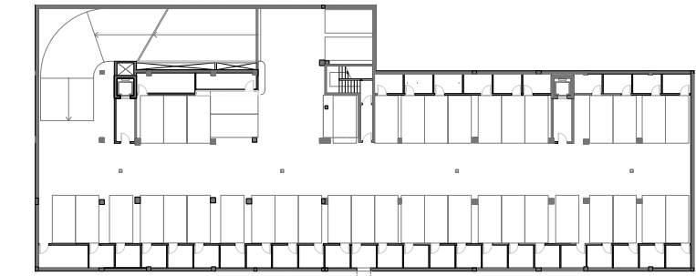
PLANTA SOTERRANI
