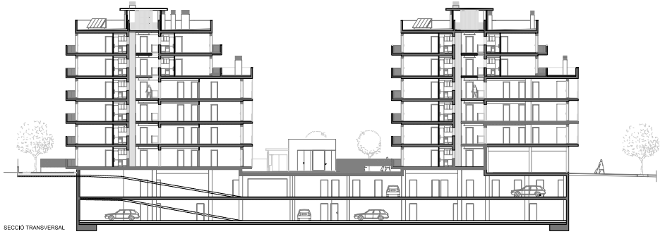
SECCIO TRANSVERSAL
