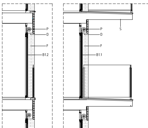
SECCIÓ S01
