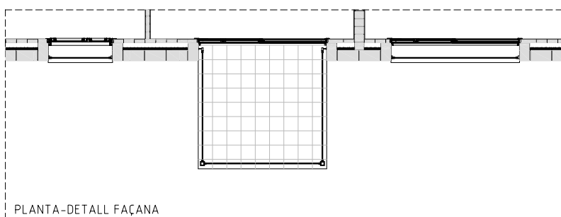
PLANTA-DETALL FAÇANA
